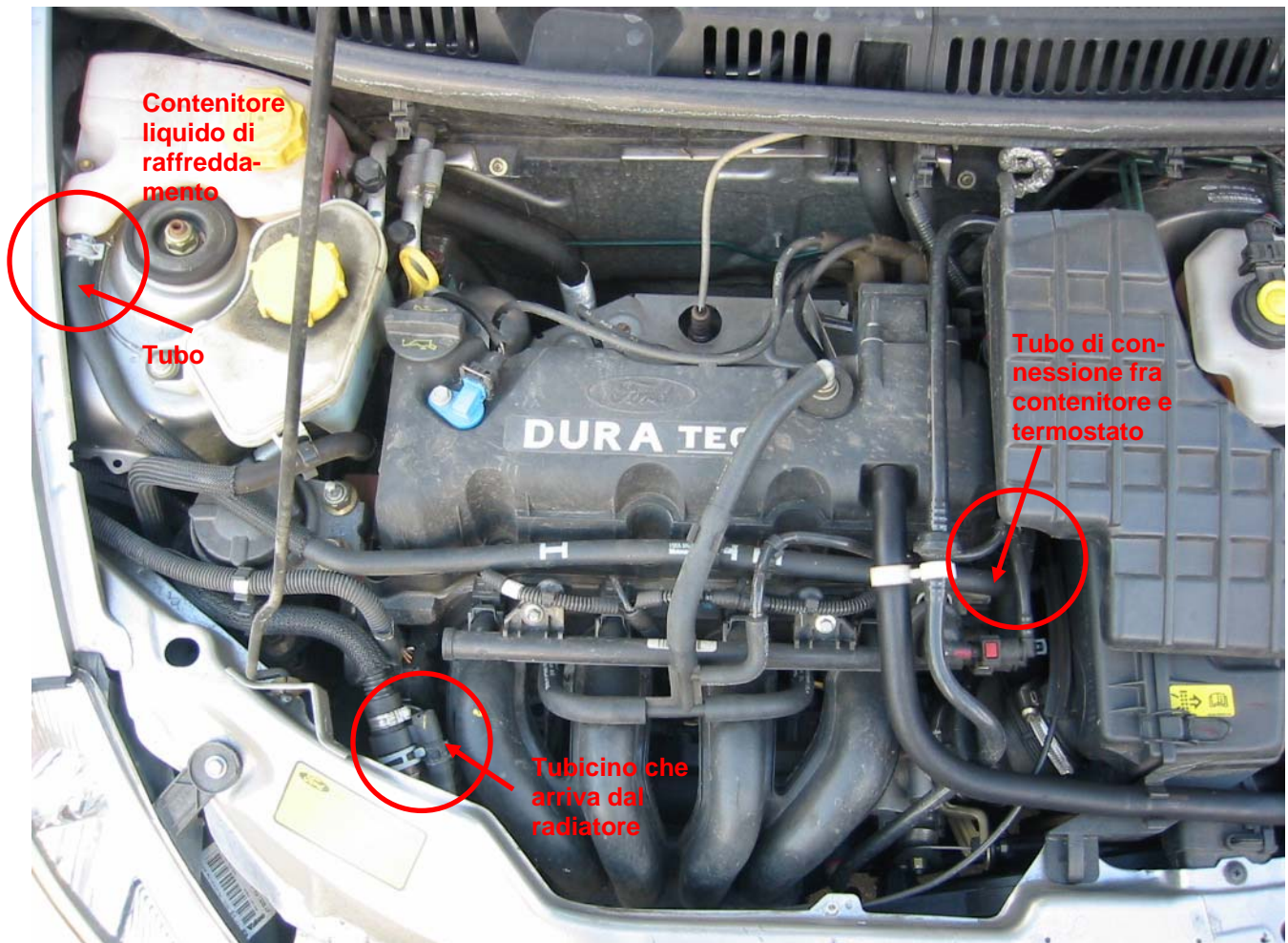
Picture 3: Comparto motore
