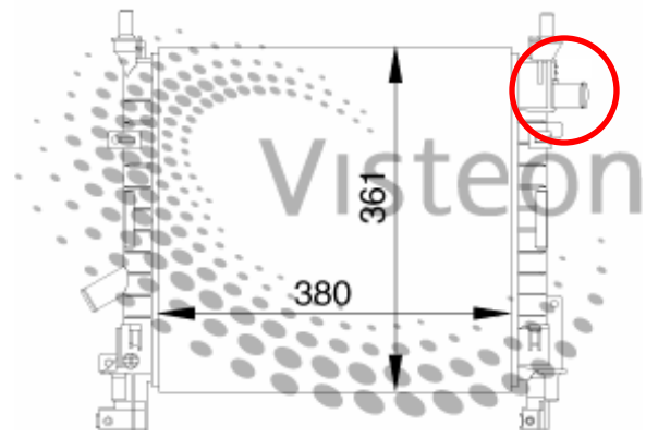
Figura 2: Radiator senza tubo (1S5H 8005 BB)
