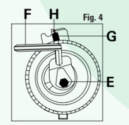
FIGURA 4 Aflojar el tornillo de fijación E del tensor de correa. Actuando con la llave hexagonal F sobre el excéntrico de regulación, girar el tensor de la correa en sentido de las agujas del reloj hasta que el indicador G y la marca H estén alineados. Por último, apriete el tornillo de fijación del tensor.
