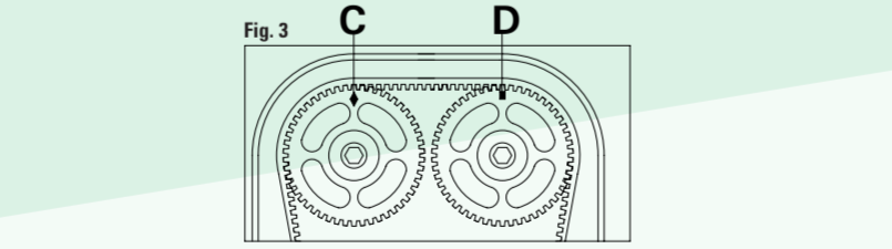
FIGURA 1 Verificar la correcta alineación de los arboles de leva A. FIGURA 2 Verificar el posicionamiento correcto la herramienta de inmovilización de árbol de levas B. FIGURA 3 Verificar el posicionamiento correcto de las marcas de fase C y D.
