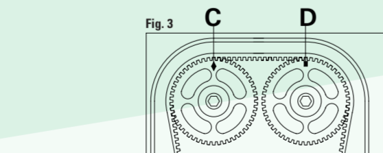
FIGURA 1 Controllare il corretto allineamento degli alberi a camme A. FIGURA 2 Controllare il corretto posizionamento dell'attrezzo di bloccaggio degli alberi a camme B. FIGURA 3 Controllare il corretto posizionamento delle tacche di fase C e D.
