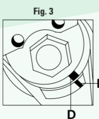
FIGURA 2 Allentare il bullone di bloccaggio B e ruotare in senso orario il tendicinghia utilizzando la chiave C agendo sull'eccentrico di registro. FIGURA 3 Allineare l'indicatore D del tendicinghia con la tacca E; serrare quindi il bullone di bloccaggio B. FIGURA 4 Allentare il bullone di bloccaggio F del tendicinghia e ruotare quest'ultimo in senso orario fino ad allineare l'indicatore G con la zona di controllo H.
