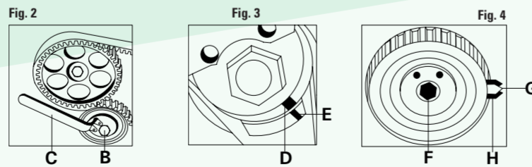
FIGURA 2 Aflojar el tornillo de fijación B, girar el tensor de correa sobre el excéntrico en sentido de las agujas del reloj, utilizando la llave de regulación C. FIGURA 3 Alinear el indicador D del tensor de la correa con la muesca E. Finalmente, apretar el tornillo de fijación B. FIGURA 4 Aflojar el tornillo de fijación F del tensor de correa. Girar el tensor de correa en sentido de las agujas del reloj hasta alinear la marca G con la zona de control H.
