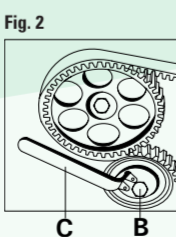
FIGURA 2 Allentare il bullone di bloccaggio B e ruotare in senso orario il tendicinghia utilizzando la chiave C agendo sull'eccentrico di registro. FIGURA 3 Allineare l'indicatore D del tendicinghia con la tacca E; serrare quindi il bullone di bloccaggio B. FIGURA 4 Allentare il bullone di bloccaggio F del tendicinghia e ruotare quest'ultimo in senso orario fino ad allineare l'indicatore G con la zona di controllo H.
