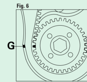
FIGURA 6 Controllare il corretto allineamento delle tacche di fase G.
